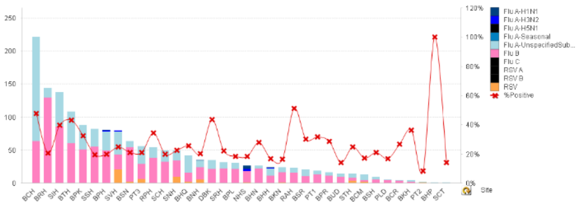
Figure 1 ผลการตรวจหาเชื้อไวรัสไข้หวัดใหญ่ จำแนกตามโรงพยาบาล จากการเฝ้าระวังทางห้องปฏิบัติการ 20 แห่ง จากกลุ่มตัวอย่างผู้ป่วย ILI ในแผนกผู้ป่วยนอกสัปดาห์ที่ 28 ระหว่างวันที่ 8 - 14 กรกฎาคม 2562
